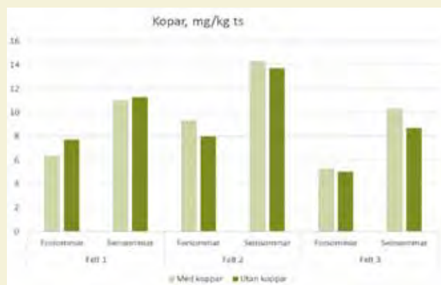
Figur 2: Innhald av kopar (mg/kg ts) i grasprøver tatt ut frå ruter gjødsla med Helgjødsel med og utan tilsetjing av kopar frå 3 forsøksfelt.
