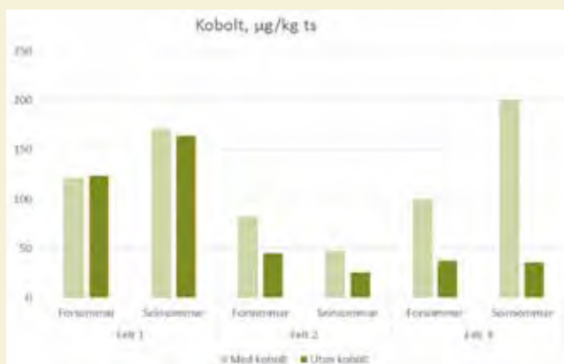
Figur 1: Innhald av kobolt (µg/kg ts) i grasprøver frå ruter gjødsla med Helgjødsel med og utan tilsetjing av kobolt frå 3 forsøksfelt.
